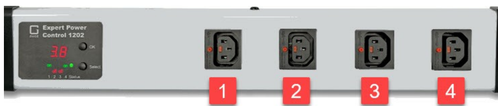
4 x Lastausgänge (IEC C13 Lock, max. 10 A) bei Expert Power Control 1202-4
