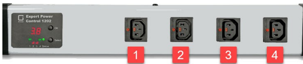
4 x Lastausgänge (IEC C13 Lock, max. 10 A) bei Expert Power Control 1202-4 / 1292-4
