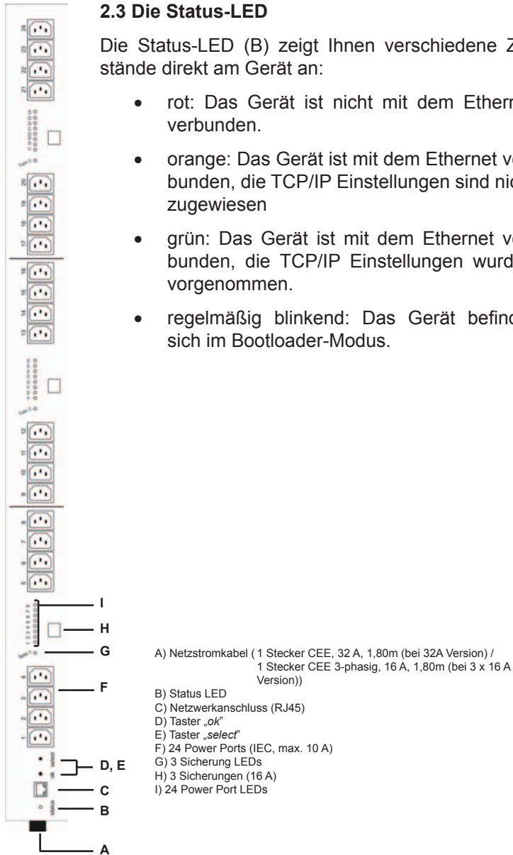
Abb. 1 Front des EPC NET 24x
